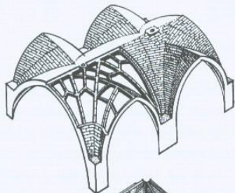
Hvězdová klenba - axonometrie
