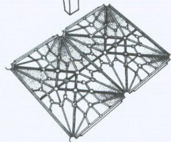
Síťová klenba - kamenný žebrový skelet s cihelnou výplní
