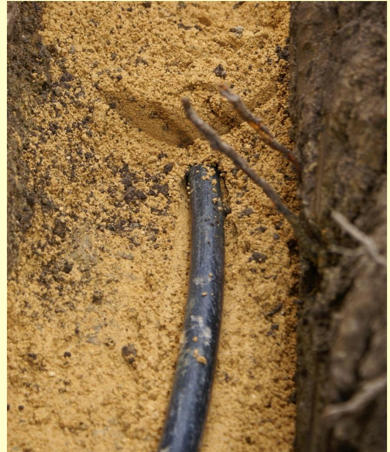
Písková vrstva nad kabelem o tl. 8 cm
